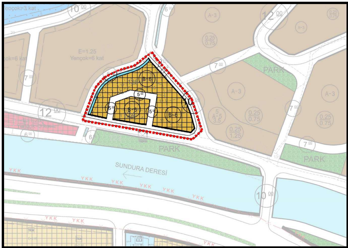
Şekil 7.1/1000 Ölçekli Uygulama İmar Planı Değişikliği
